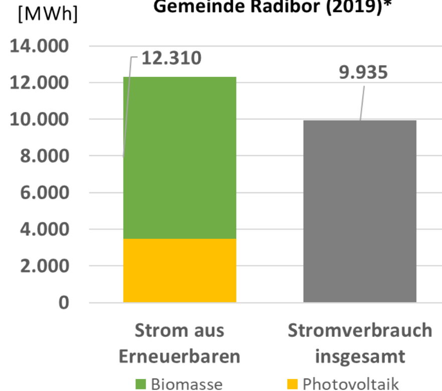
Stromerzeugung und Strombedarf in der Gemeinde Radibor (2019)*
